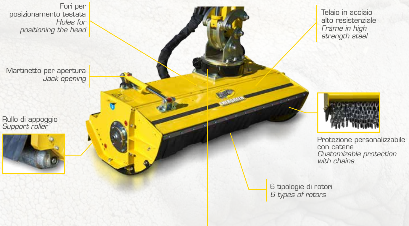
Ralla con rotazione di 180° Slewing bearing 180° rotation
